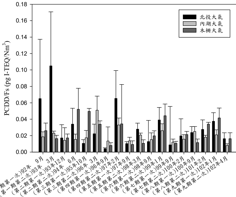
圖 A01 第一至九期臺北市三座焚化廠大氣 PCDD/Fs 檢測結果比較
