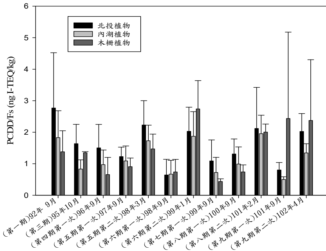
圖 A01 第一至九期臺北市三座焚化廠大氣 PCDD/Fs 檢測結果比較
