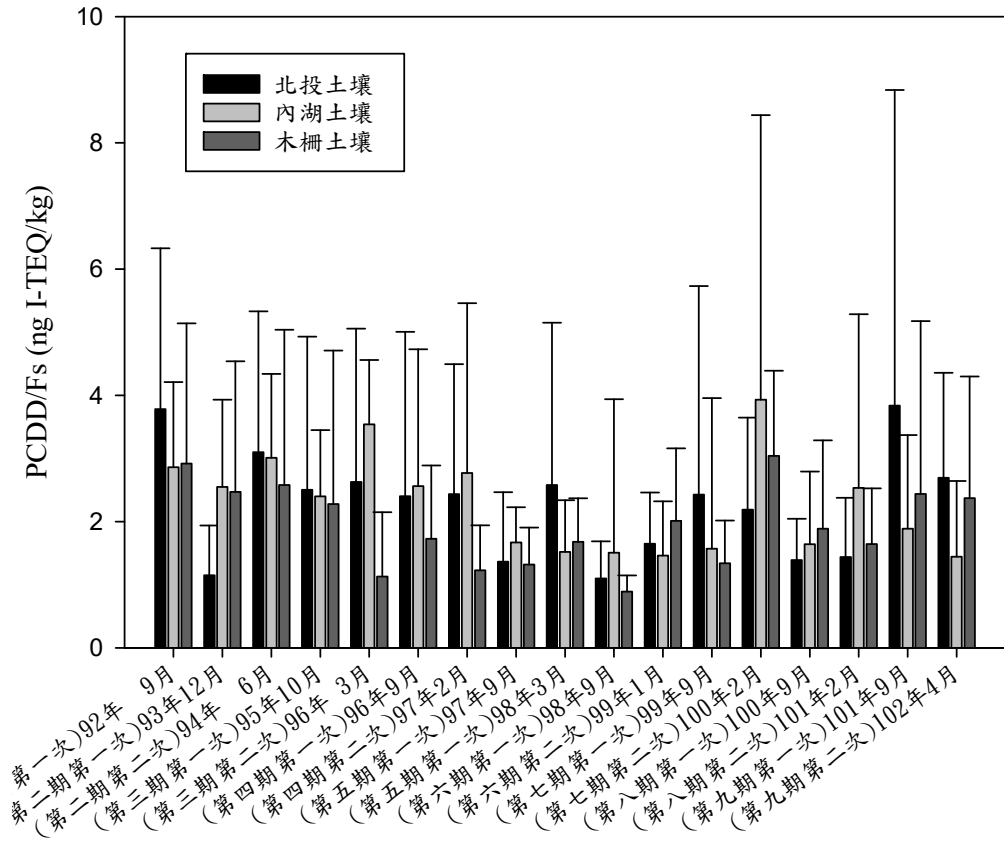
圖 A03 第一至九期臺北市三座焚化廠土壤 PCDD/Fs 檢測結果比較
