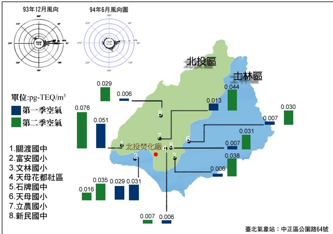
北投廠周界空氣戴奧辛濃度分析結果示意圖93.12.13~93.12.15
